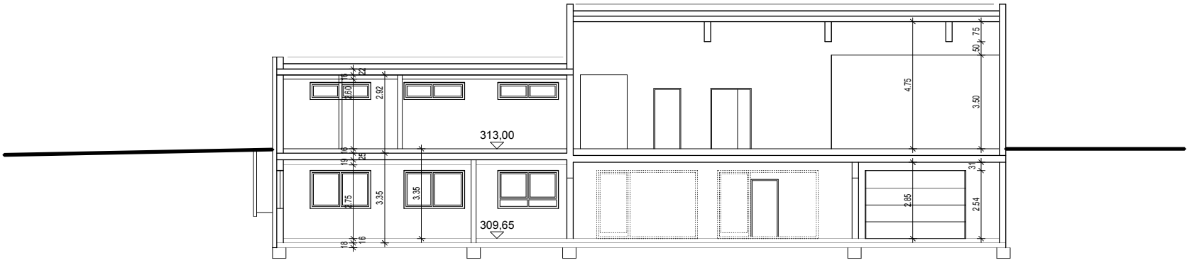
SYSTEMSCHNITT
