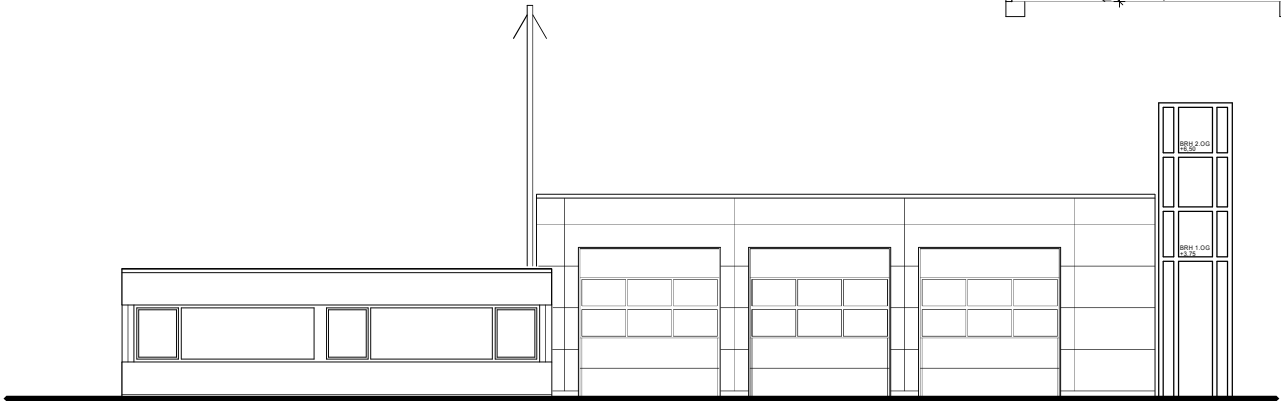
ANSICHT SÜDOST
