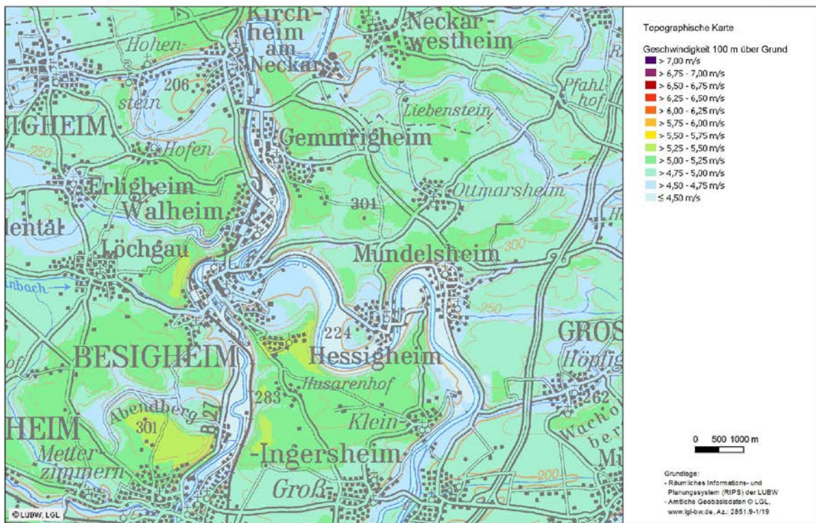
Windgeschwindigkeiten
