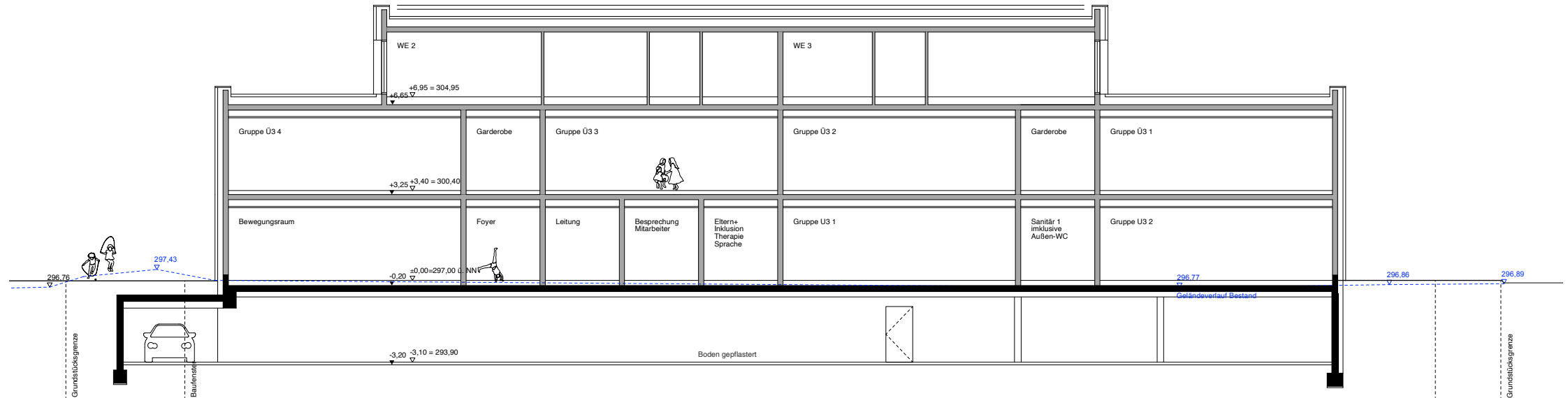
Schnitt A-A
